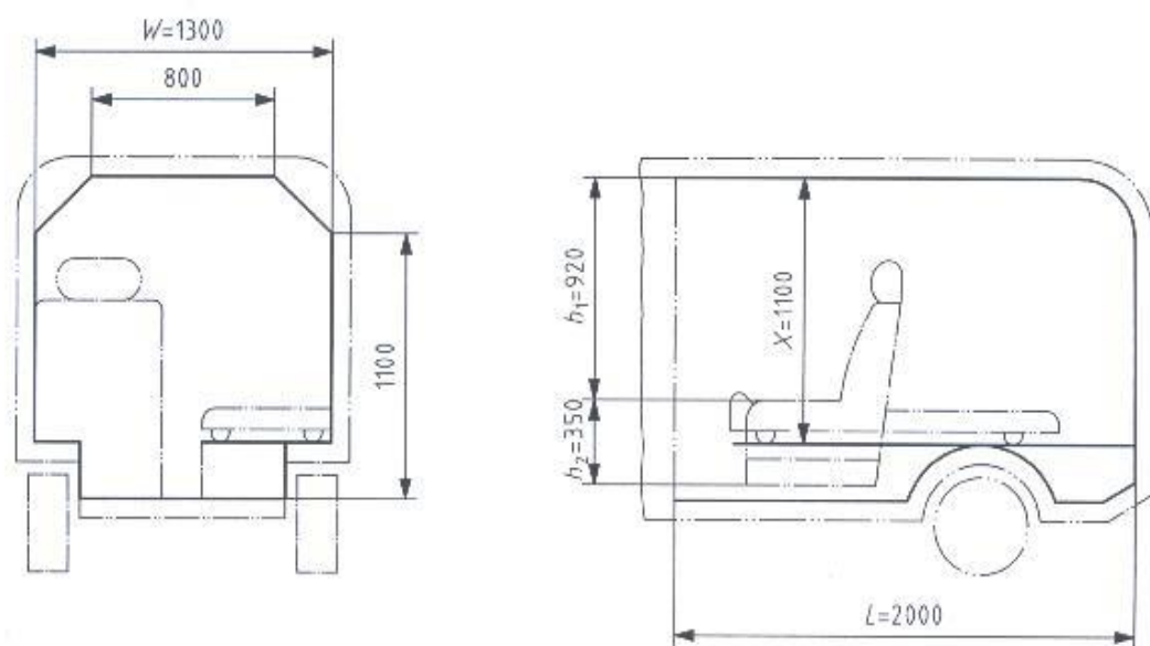
شکل ۲- شمایی از ابعاد کابین بیمار برای آمبولانس نوع A ۱
